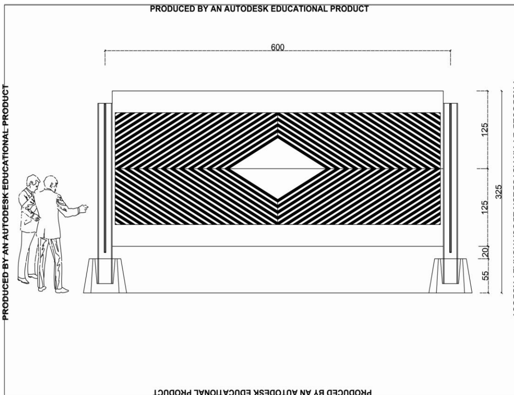
۵- دیوار بتنی به ابعاد طول ۶ متر و ارتفاع ۳,۲۵ متر و ضخامت دیوار ۱۲ سانتیمتر طرح لوزی کشویی
